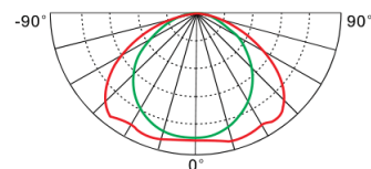
配光曲線
